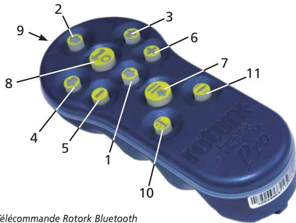
Fig 7.4 Télécommande Rotork Bluetooth
