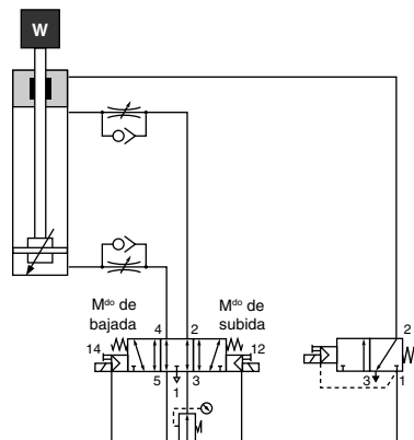
Fig. 4 - Carga sobre el cilindro.
